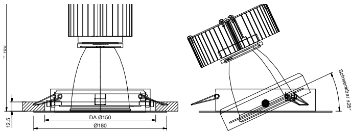
Skizze für 2x25°. Die Höhe ist abhängig vom Reflektor! Sketch for 2x25°. The height depends on the reflector!
